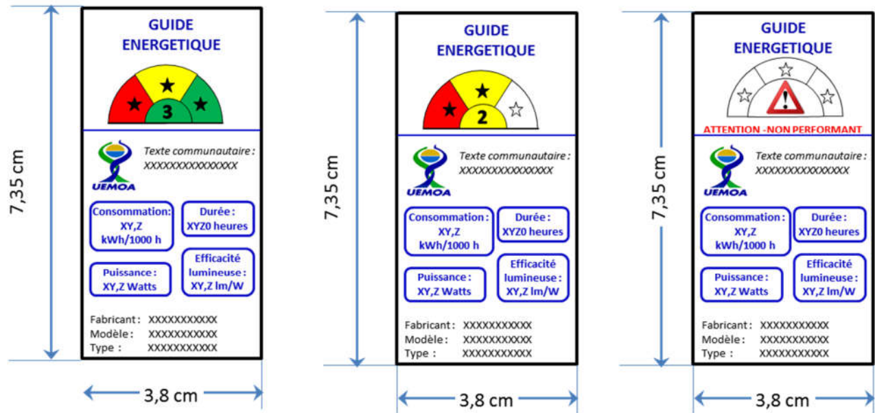
Figure 1 : Modèle d'étiquette énergétique des lampes
